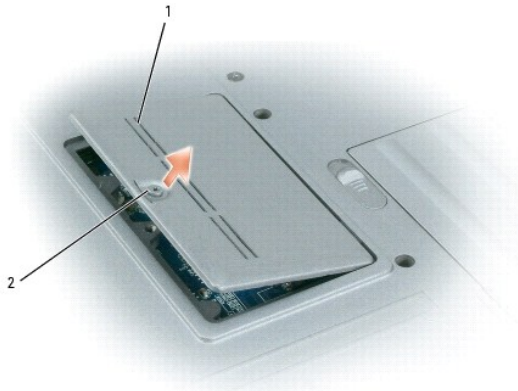
1 記憶體模組護蓋 2 緊固螺絲
