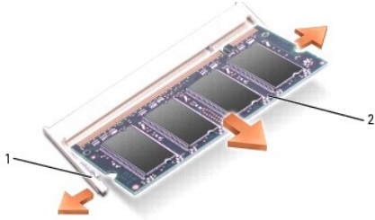
1 固定夾 (每個連接器 2 個) 2 記憶體模組
